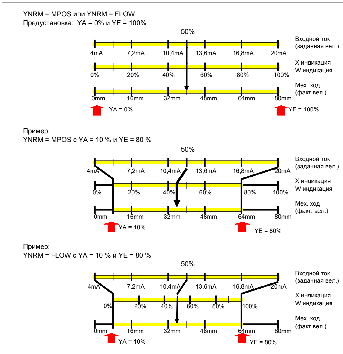
Рис. 4-9 Зависимость хода от нормирования, а также от YA и YE на примере 80 мм-поступательного привода
