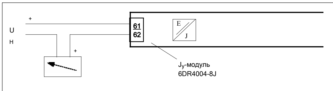
Рис. 3-17 J y -модуль 6DR4004-8J, без Ex
