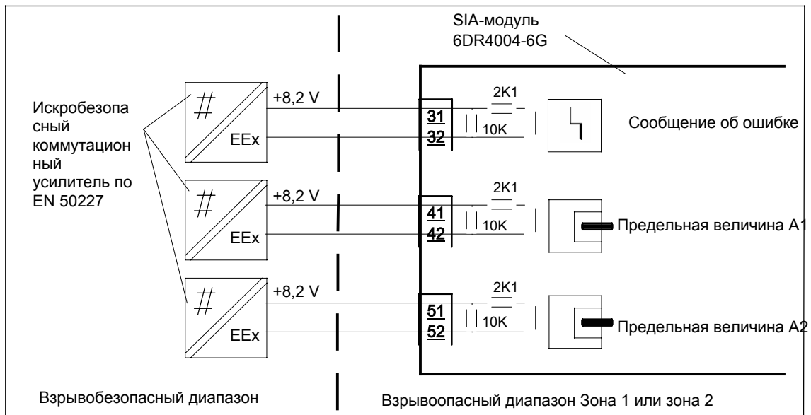
Рис. 3-22 SIA-модуль 6DR4004-8G, Ex
