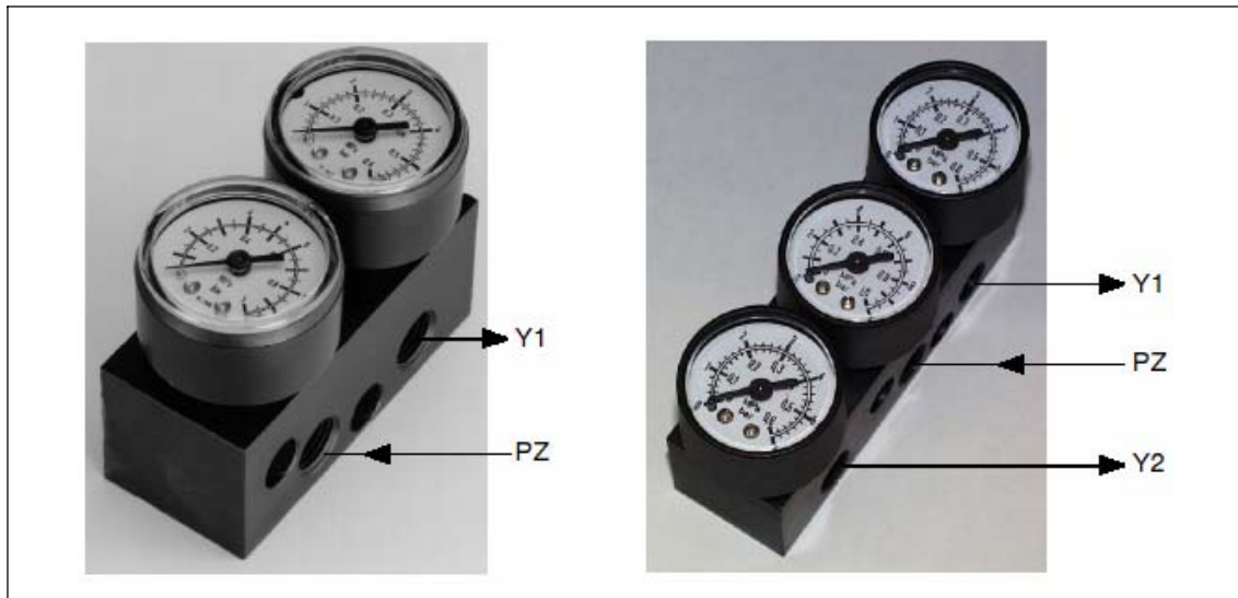
Рис. 2-12 Блок манометров (слева для приводов простого действия, справа для приводов двойного действия)
