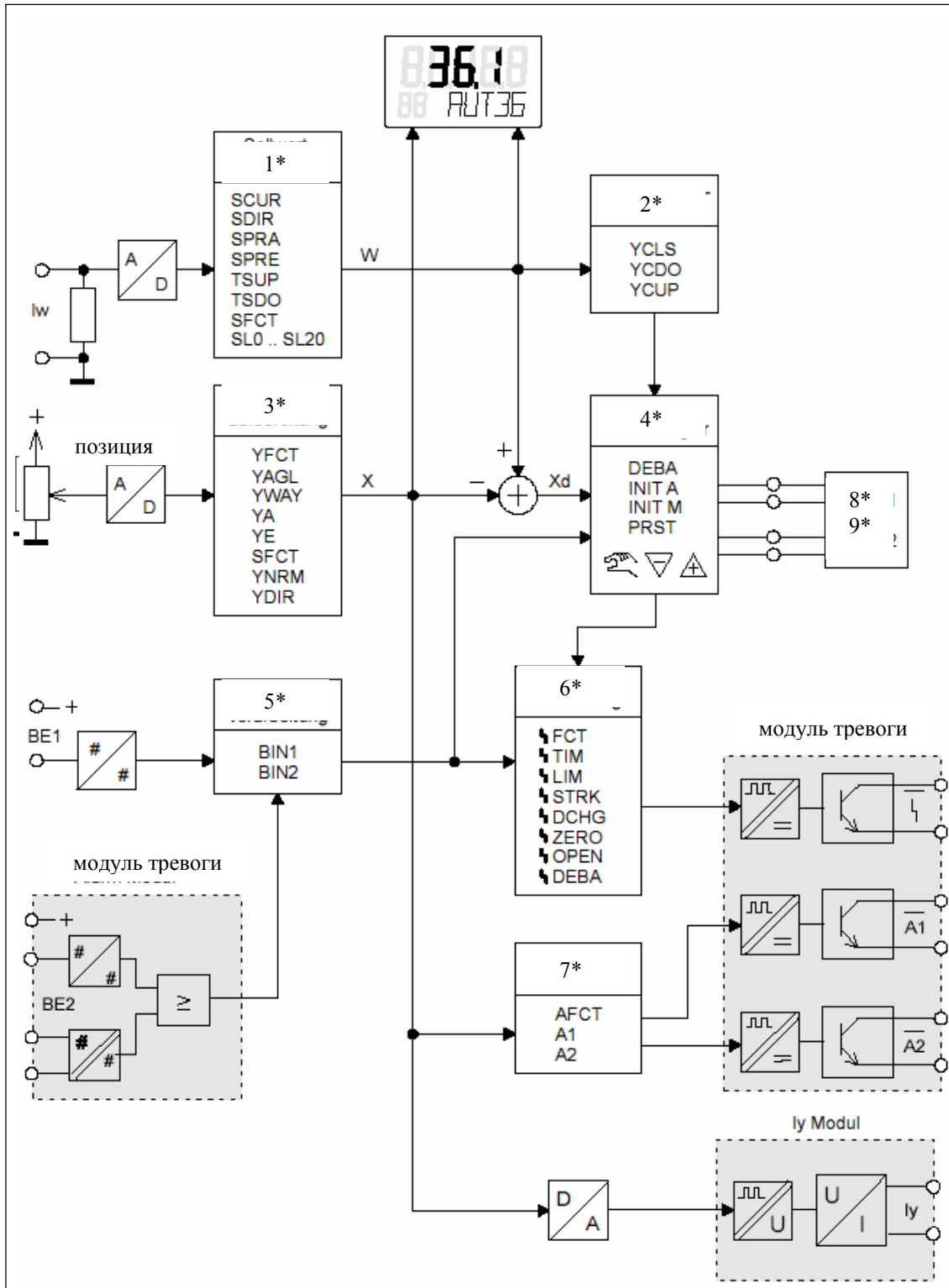
Рис. 4-10 Блок-схема конфигурации
