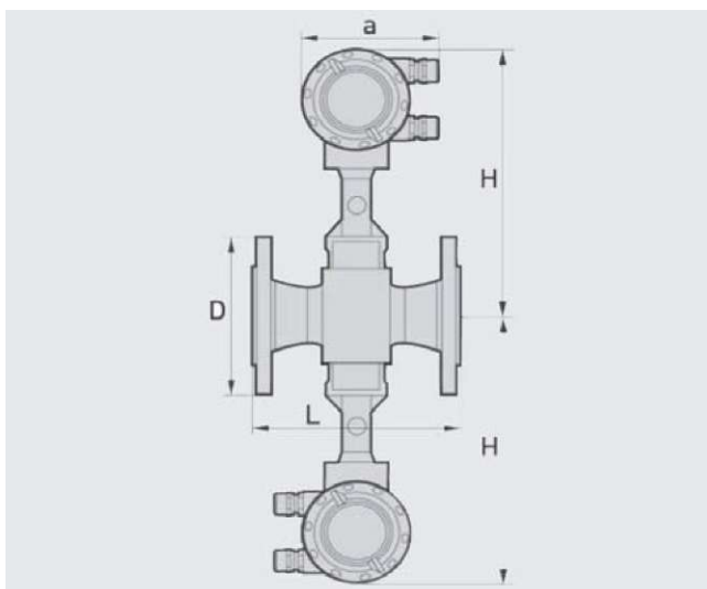
Фланцевая версия, двойной преобразователь, указанный вес + 2.80 кг
