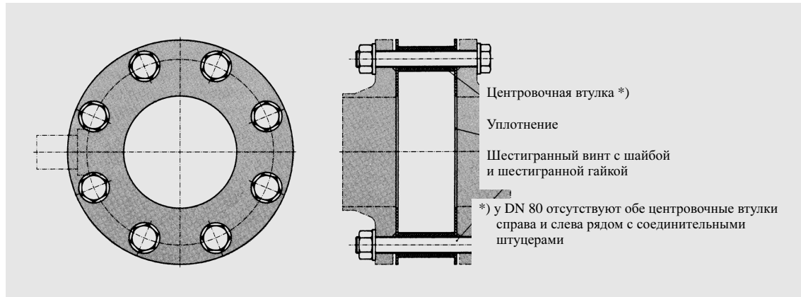
Рис 3/99 Центрировочный набор
