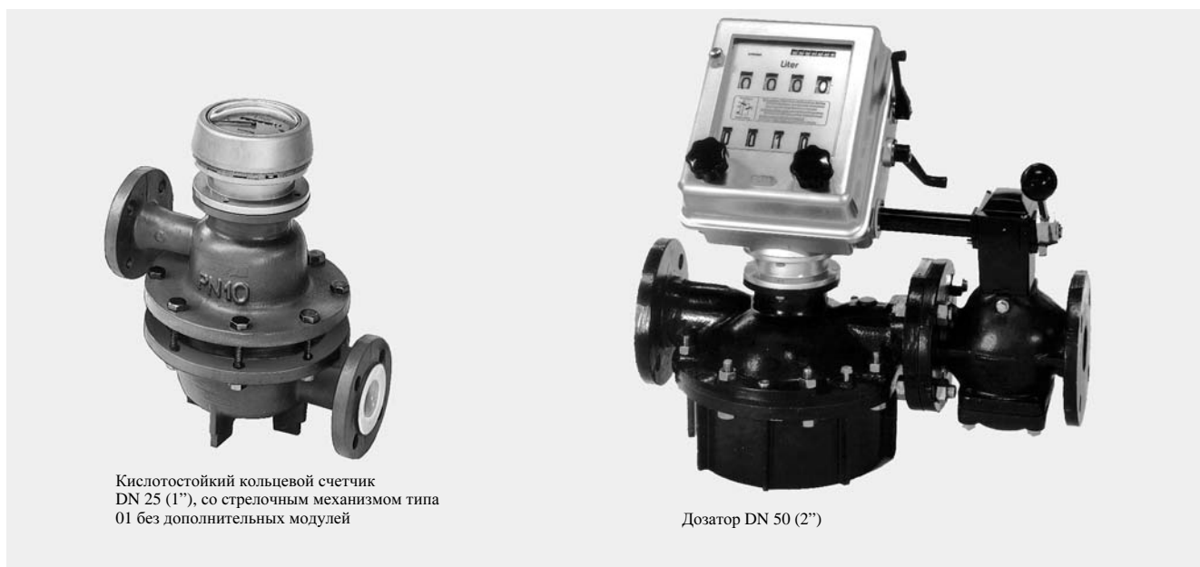
Рис 3/130 Кислотостойкий кольцевой счетчик и дозатор
