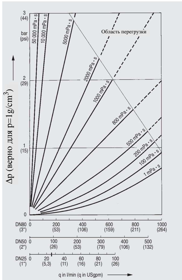
Рис 3/136 Рабочие диапазоны для кольцевых счетчиков DN 25 (1"), 50 (2") и 80 (3"); потеря давления в зависимости от протока и вязкости измеряемого вещества
